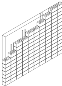
Muros de carga de mampostería
